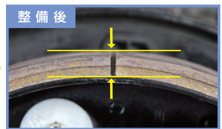
ブレーキ・シュー(ライニング)が新品の状態
